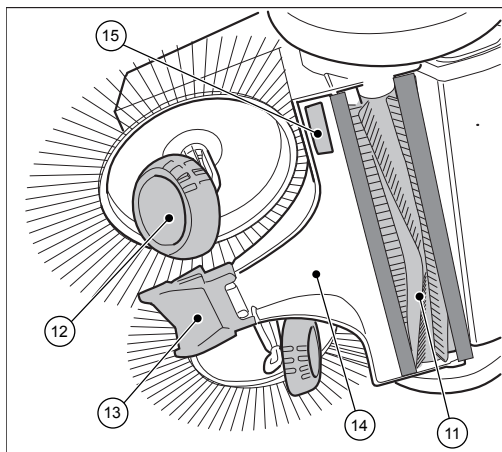
Kuva 2: Laitteen osat 2
