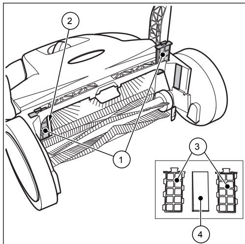
Kuva 12: Pölynsuodattimen poistaminen
