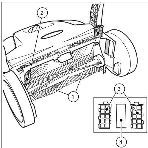
Fig. 12: Å ta ut støvfiltre
