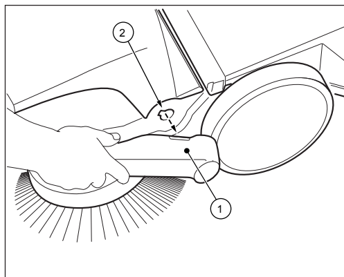
Bild 14: Nedmontering av skjutbygel (inte haaga 375)
