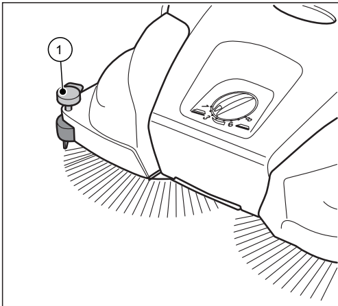
Abb. 10: Niederhalterereinstellung Auskehren von Kanten und Ecken
