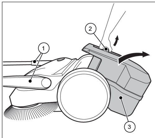
Рис. 11: Опорожнение бункера
