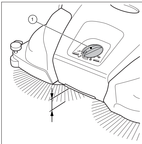
Abb. 9: Höhenverstellung Tellerbesen
