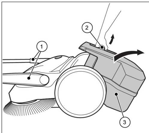
Fig. 11: Affaldsbeholderen tømme
