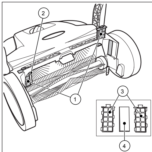
Afb. 12: Stoffilter verwijderen
