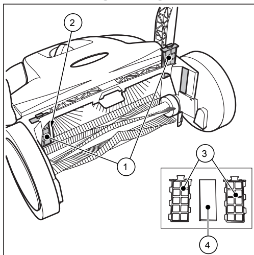
Fig. 12: Støvfilter fjernelse
