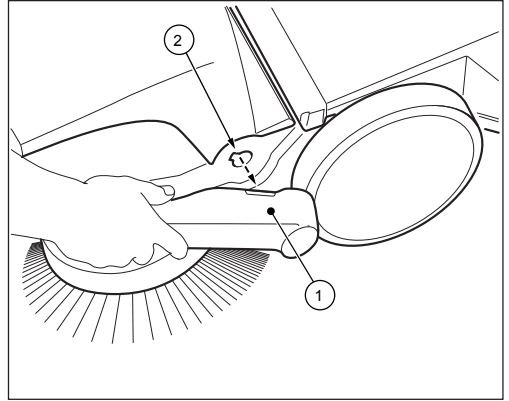
Şek. 14: İtme kolunun söküm işlemi (haaga 375 değil)
