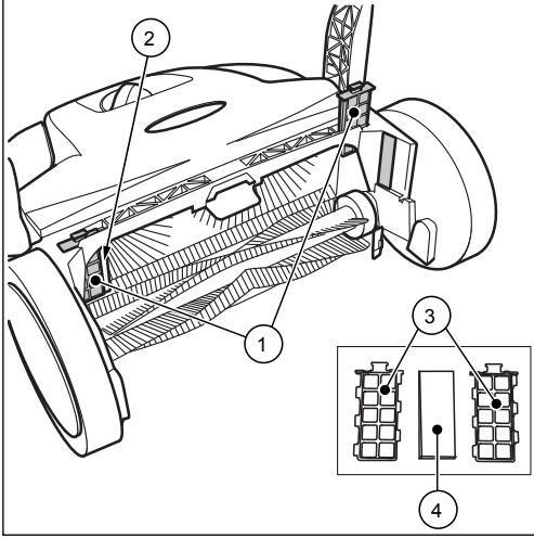
Şek. 12: Toz filtresinin çıkartılması
