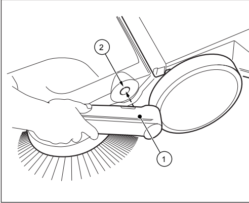
Şek. 7: Tutacak parçalarının montaj işlemi (haaga 375)
